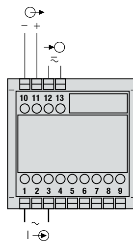
Fig. 5. Pour mesure avec 2ème (supérieure) étendue de mesure, alimentation auxiliaire à basse tension sur bornes 12 et 13.
