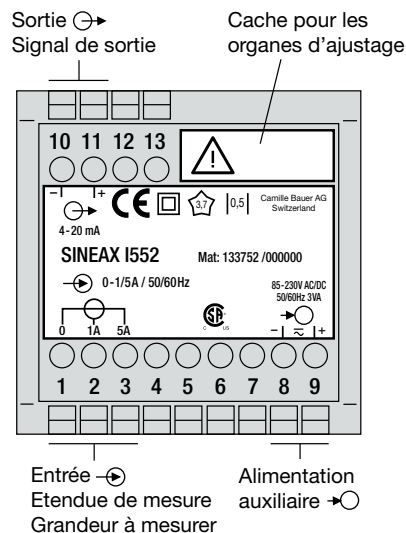
Fig. 6. Explication des inscriptions sur la plaquette signalétique.
