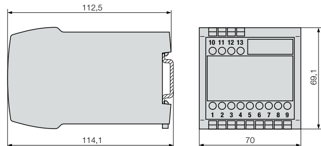
Fig. 9. Boîtier type P13/70 encliqueté sur rail «à chapeau» (35 x 15 mm ou 35x7,5 mm, selon EN 50 022).
